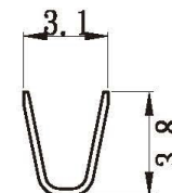
A-A Section
